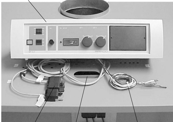
Brennerstecker Verkleidungsöffnung Kapillarrohre
