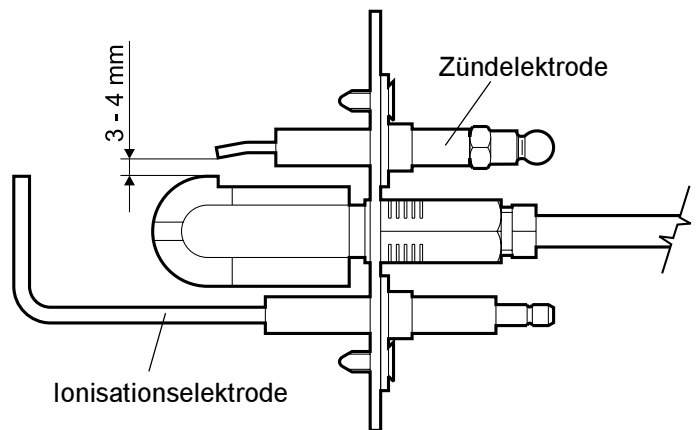
Abb. 10.3 Zündeinrichtung
