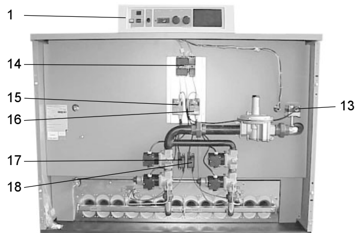
Abb. 2.2 Elektrokompnenten GA 220/119-221 E
