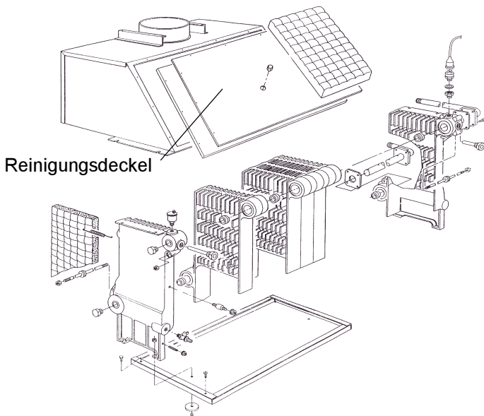
Abb. 10.2 Wärmetauscher
