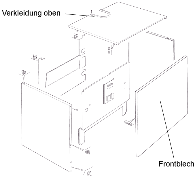
Abb. 10.1 Kesselverkleidung
