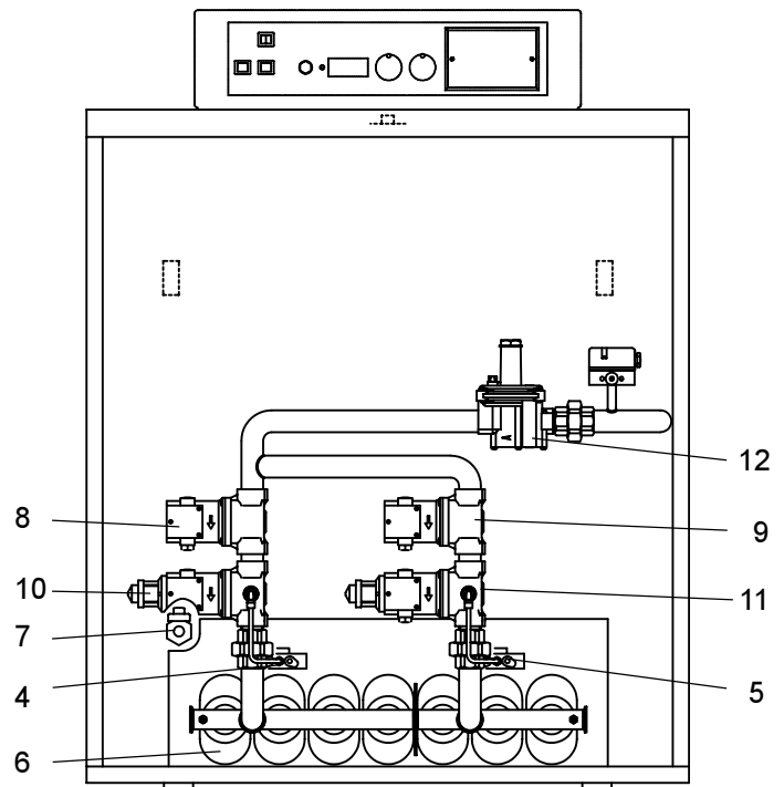
Abb. 2.1 Gas- und Brennerkomponenten GA 220/119-221 E
