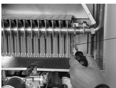
Befestigungsschrauben
