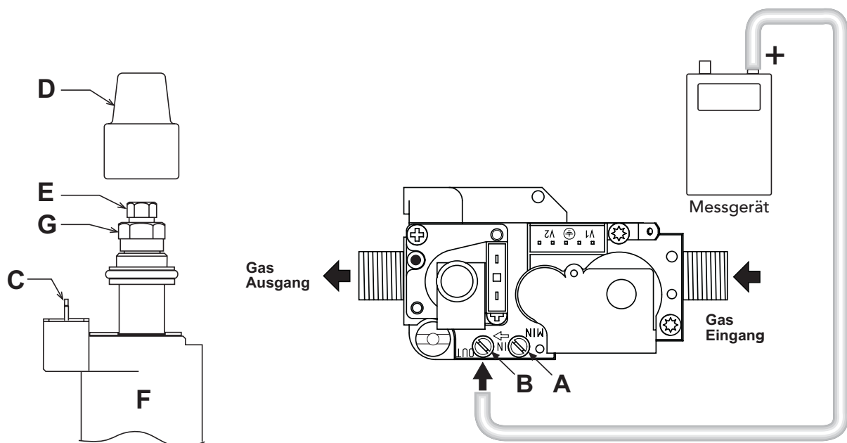
Abb. 33 - Gasventil
