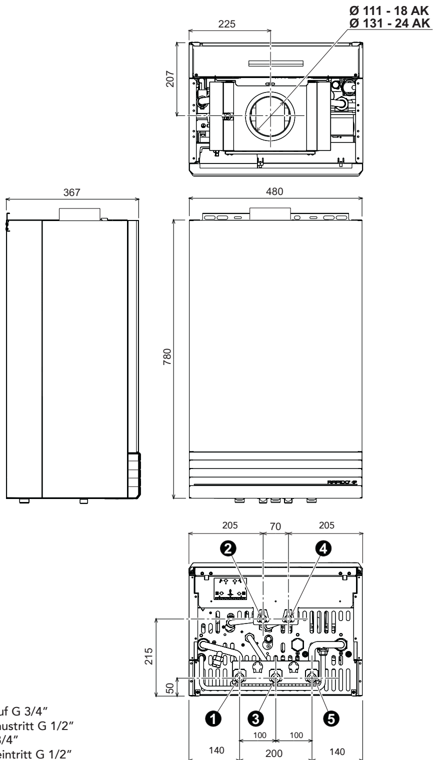
Abb. 35 - Abmessungen und Anschlüsse
