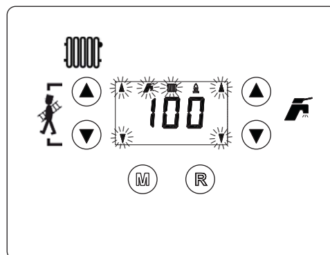
Abb. 32 - TESTBETRIEB (Heizleistung = 100%)
