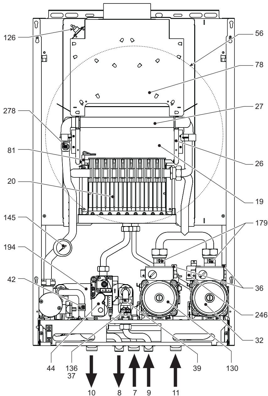
Abb. 36 – Gesamtansicht
