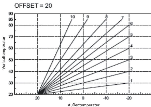
Abb. 14 - Beispiel für die Parallelverschiebung der Heizkurven
