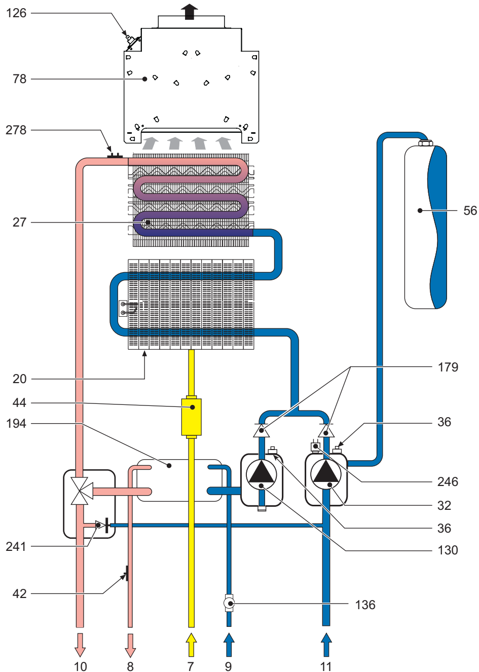
Abb. 37 - Wasserkreis
