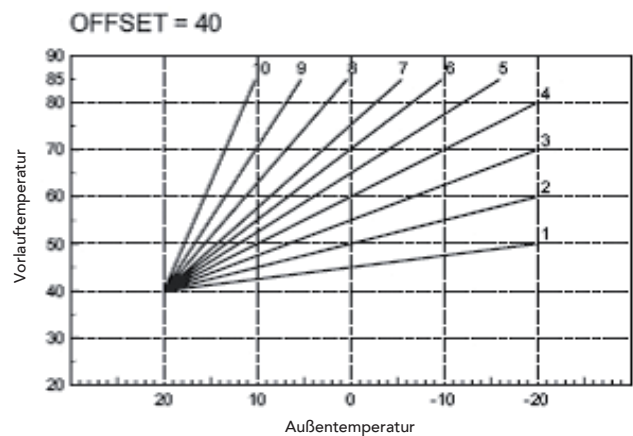
Abb. 14 - Beispiel für die Parallelverschiebung der Heizkurven
