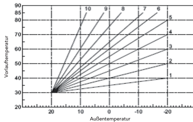
Abb. 13 - Heizkurven
