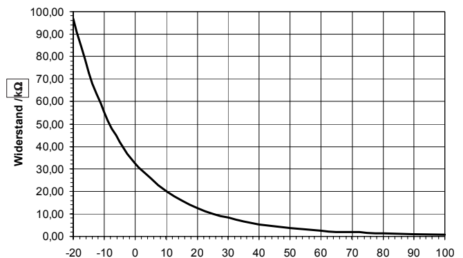
Abb. 4.23 Widerstandswerte Temperatur / °C
