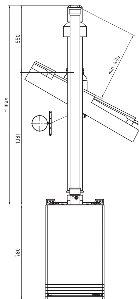
Abb. 4.12 Abgasführung senkrecht über Dach
