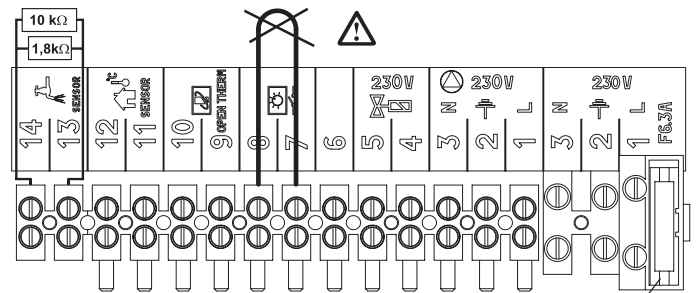
Abb. 4.19 Klemmleiste
