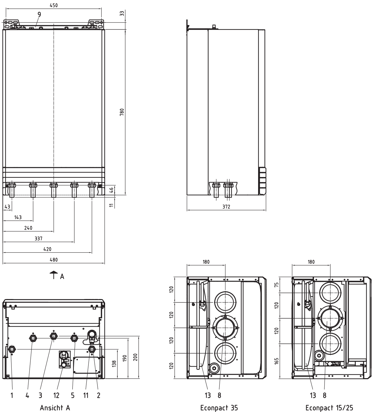
Abb. 2.4 Geräteabmessungen Econcompact 15/ 25/ 35
