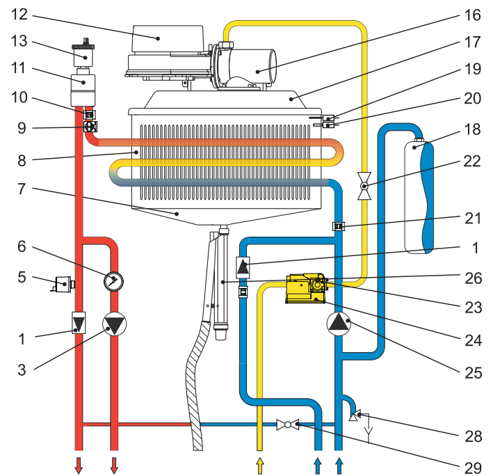
Abb. 2.2 Schema des Wärmezeugers
