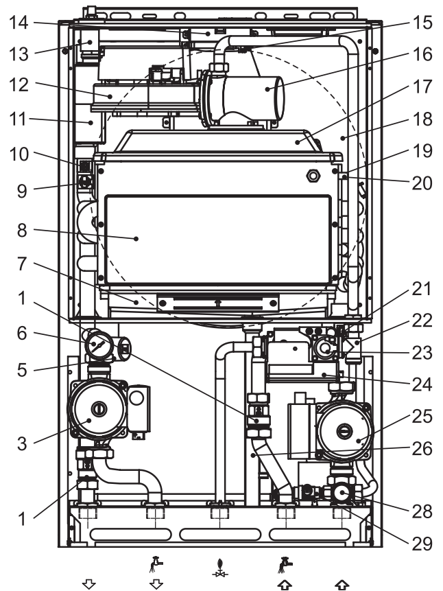
Abb. 2.1 Wärme erzeugereinheit
