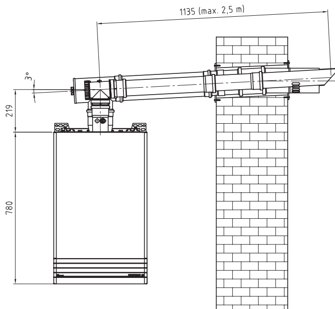
Abb. 4.11 Raumluftunabhängiger Außenwandanschluß
