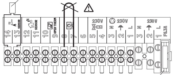
Abb. 4.27 Klemmleiste
