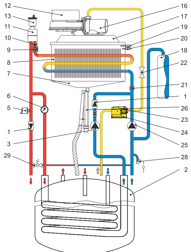
Abb. 2.2 Schema des Wärmeerzeugers
