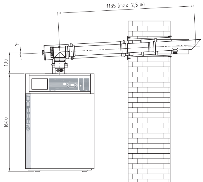
Abb. 4.21 Raumluftunabhängiger Außenwandanschluß
