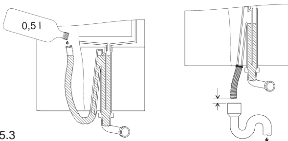
Kondensatschlauch
