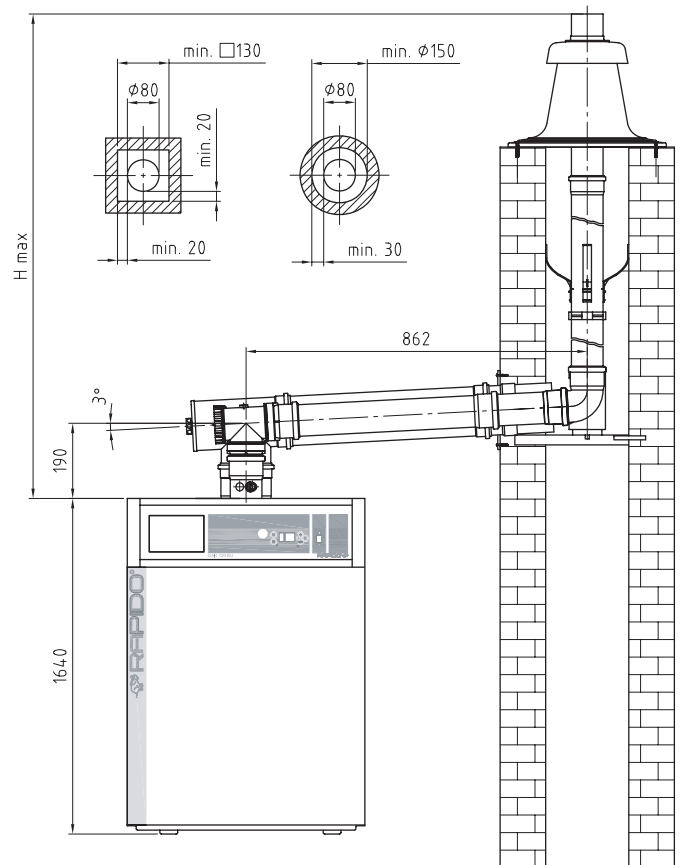
Abb. 4.19 Raumluftunabhängige Abgasführung im Schacht
