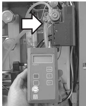
Abb. 5.12 Gasdruckmessung
