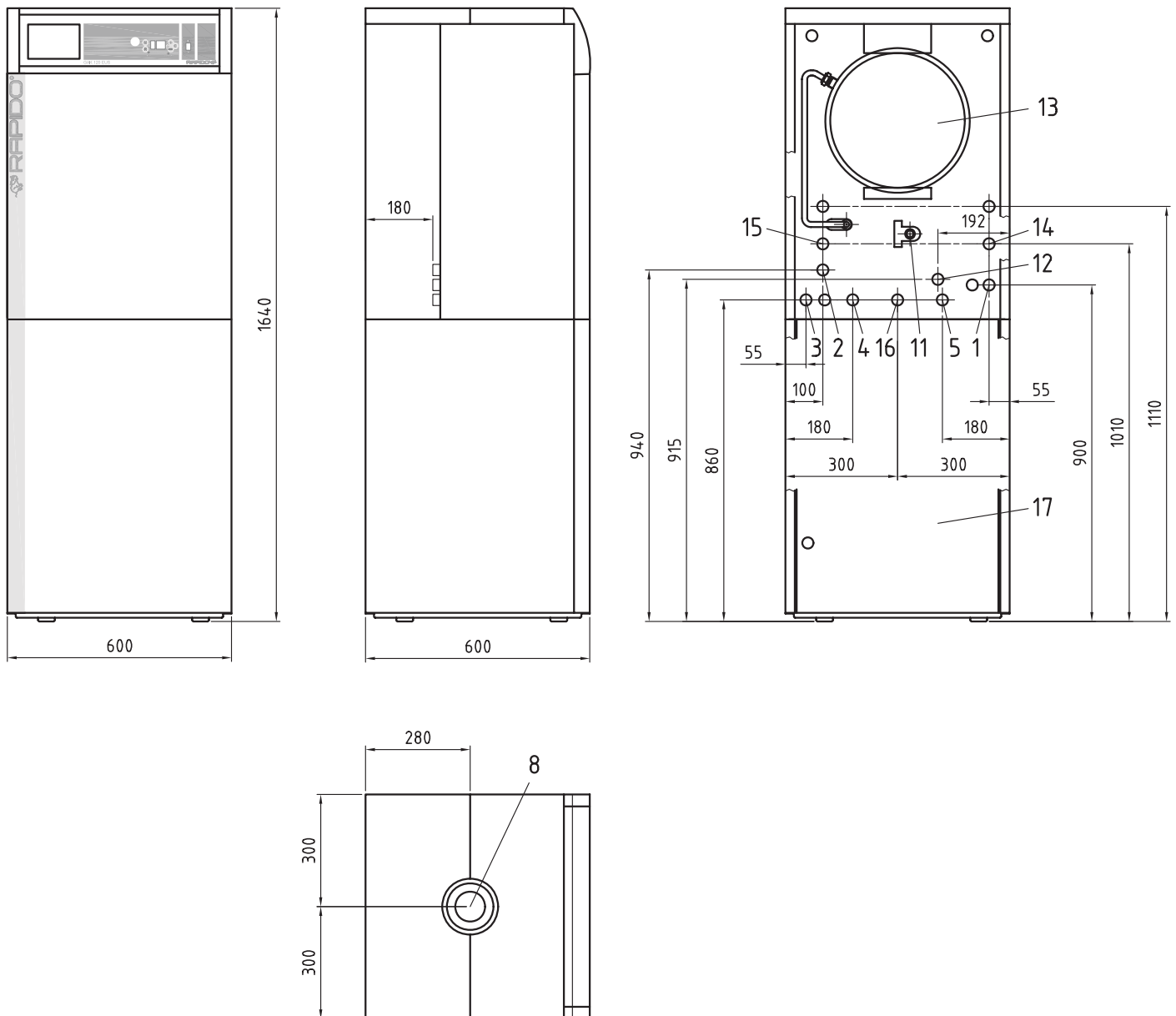
Abb. 2.4 Geräteabmessungen Econfloor GAK 15/ 25 EUS
