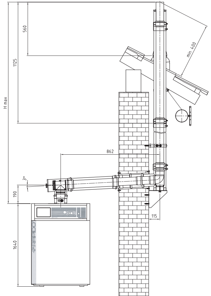
Abb. 4.24 Raumluftunabhängiger vertikaler Außenwandanschluß mit Schrägdachdurchführung
