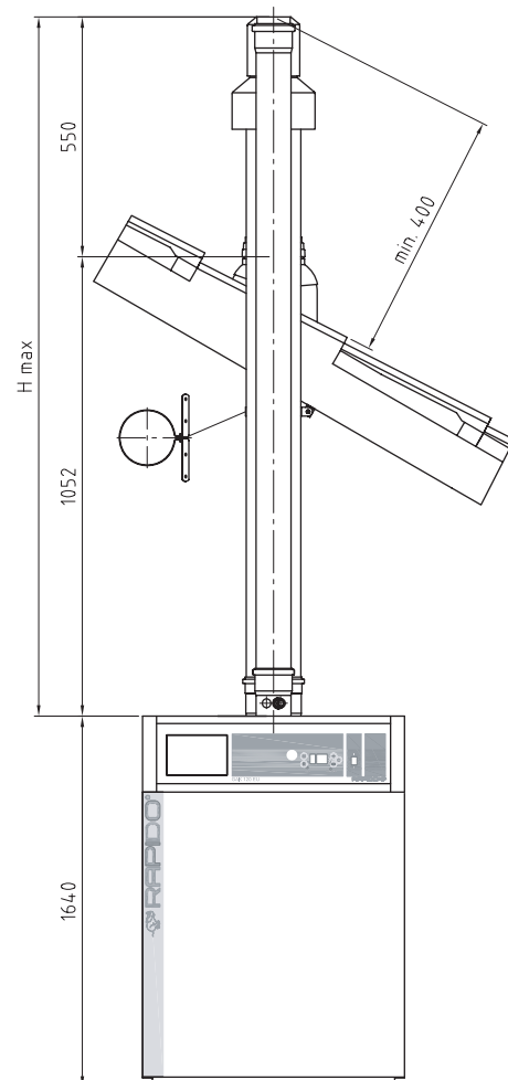
Abb. 4.22 Abgasführung senkrecht über Dach
