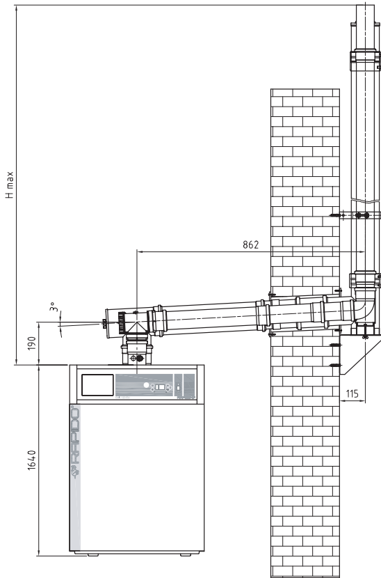
Abb. 4.23 Raumluftunabhängiger vertikaler Außenwandanschluß
