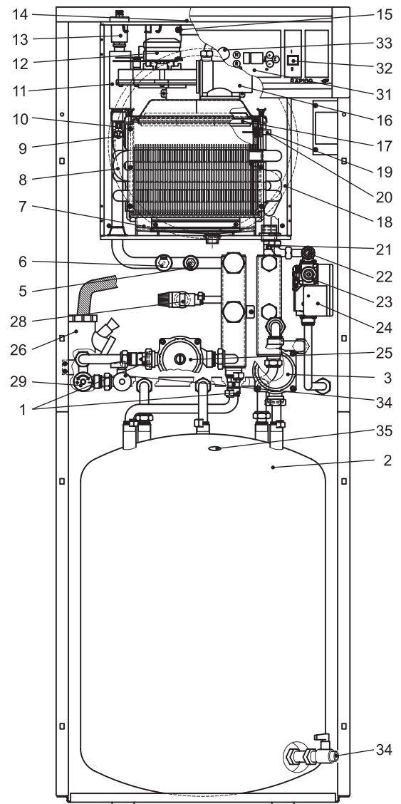
Abb. 2.1 Wärmeerzeugereinheit
