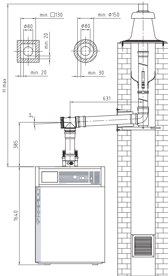
Abb. 4.20 Raumluftabhängige Abgasführung im Schacht
